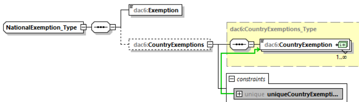
Obrázok č. 17: DAC6 National Exemption Type Diagram
