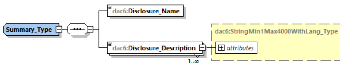
Obrázok č. 18: DAC6 summary Type Diagram
