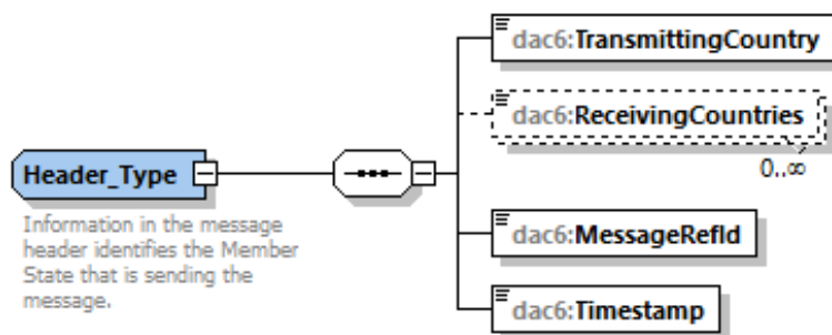
Obrázok č. 2: DAC6 Header Diagram
