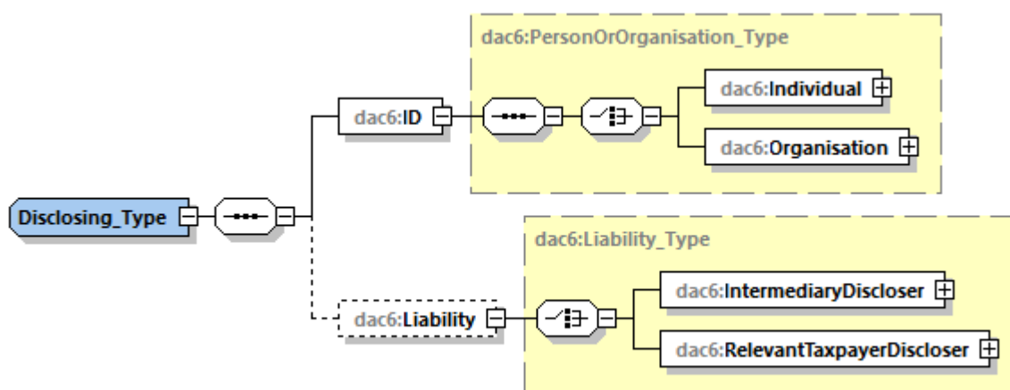
Obrázok č. 5: DAC6 Disclosing Diagram
