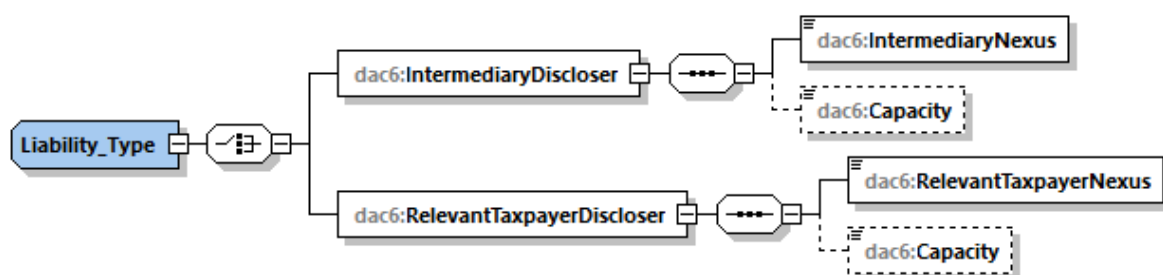
Obrázok č. 16: DAC6 Liability Type Diagram
