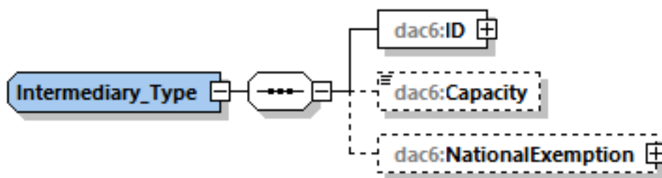
Obrázok č. 7: DAC6 Intermediary Diagram
