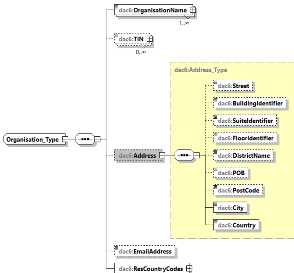
Obrázok č. 12: DAC6 Organisation Type Diagram
