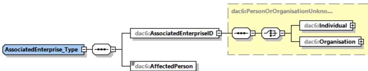
Obrázok č. 15: DAC6 Associated Enterprise Type Diagram
