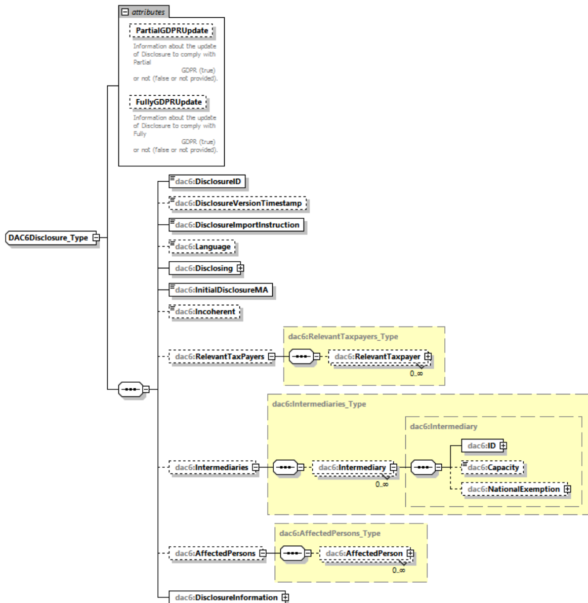
Obrázok č. 4: DAC6 Disclosure Diagram
