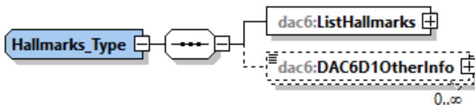
Obrázok č. 21: DAC6 Hallmarks Type Diagram
