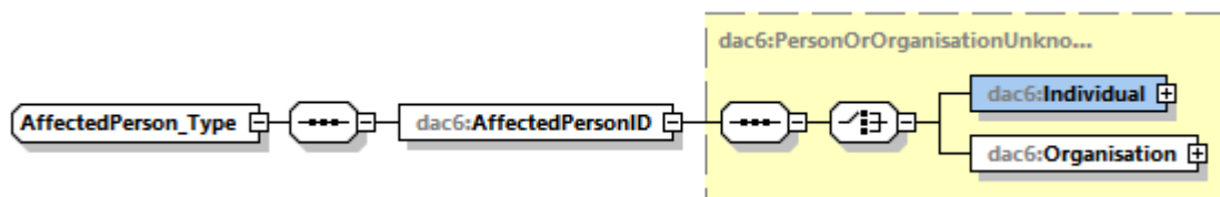
Obrázok č. 14: DAC6 Affected Person Type Diagram
