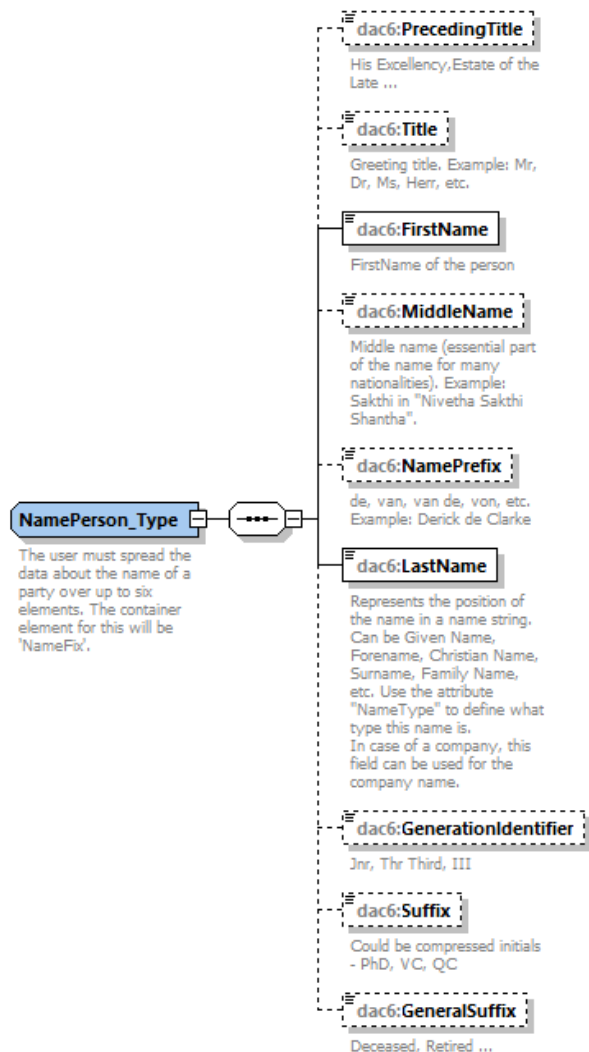
Obrázok č. 11: DAC6 NamePerson Type Diagram
