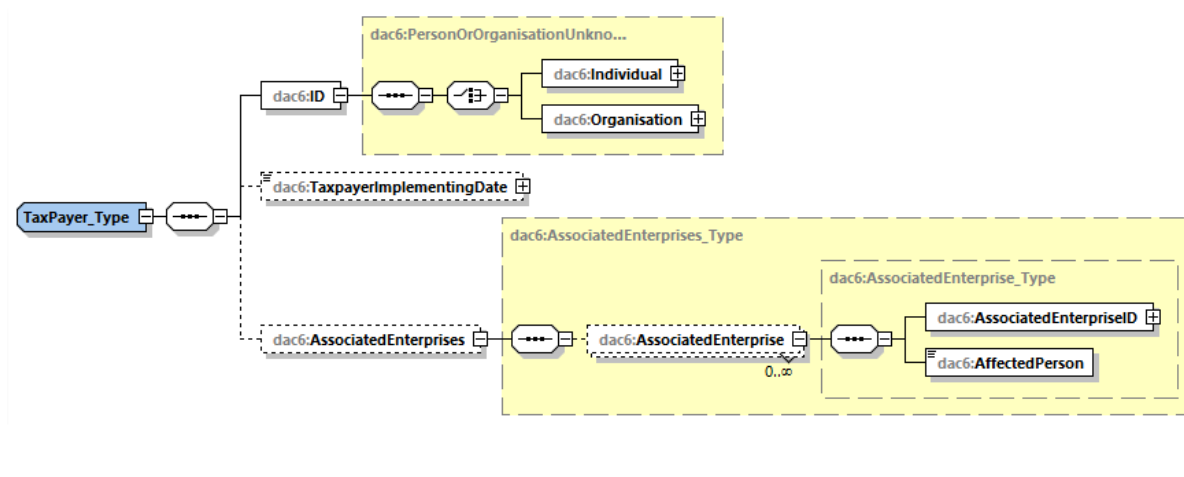
Obrázok č. 6: DAC6 Relevant Taxpayer Diagram
