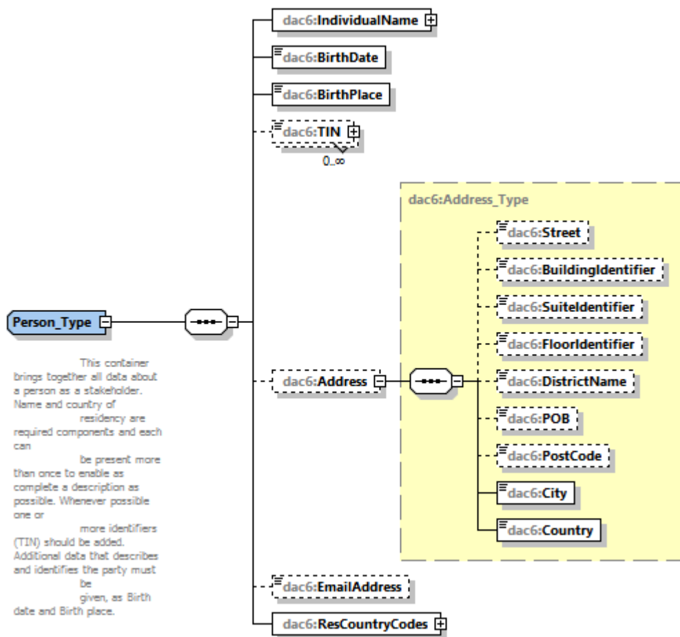
Obrázok č. 10: DAC6 Person Type Diagram
