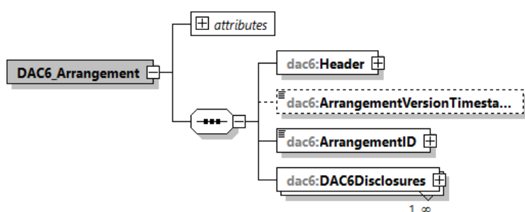
Obrázok č. 1: DAC6 Arrangement Diagram
