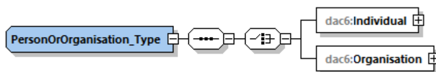
Obrázok č. 9: DAC6 Person or Organisation Type Diagram
