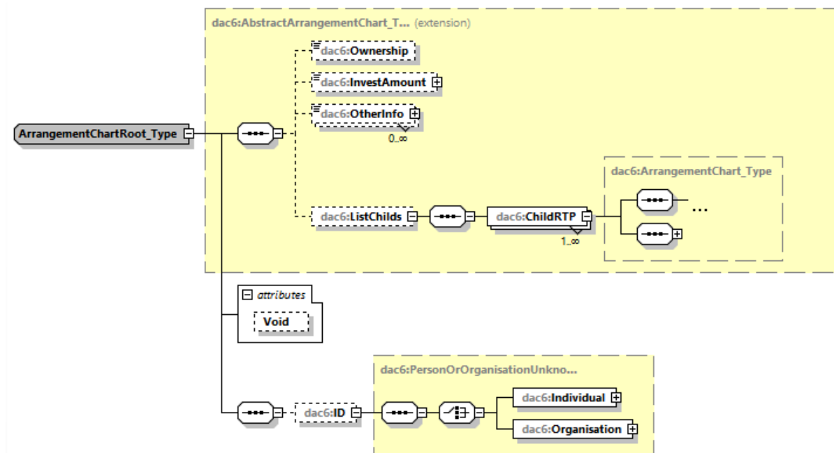
Obrázok č. 1: DAC6 Arrangement Chart Root Type Diagram
