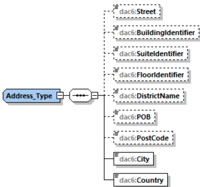
Obrázok č. 13: DAC6 Address Type Diagram
