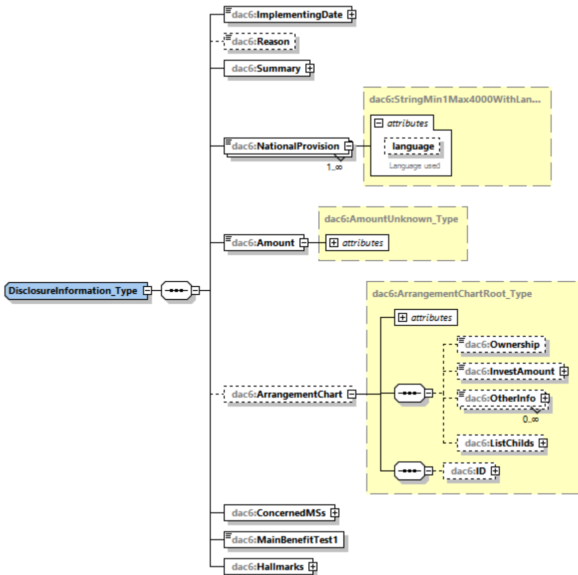
Obrázok č. 8: DAC6 Disclosure Diagram
