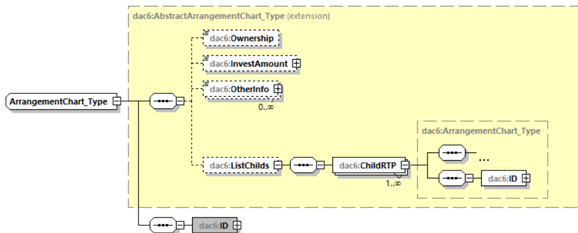
Obrázok č. 19: DAC6 Arrangement Chart Type Diagram
