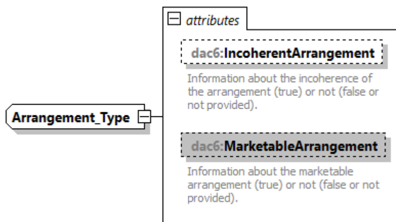
Obrázok č. 3: DAC6 Arrangement Type Diagram
