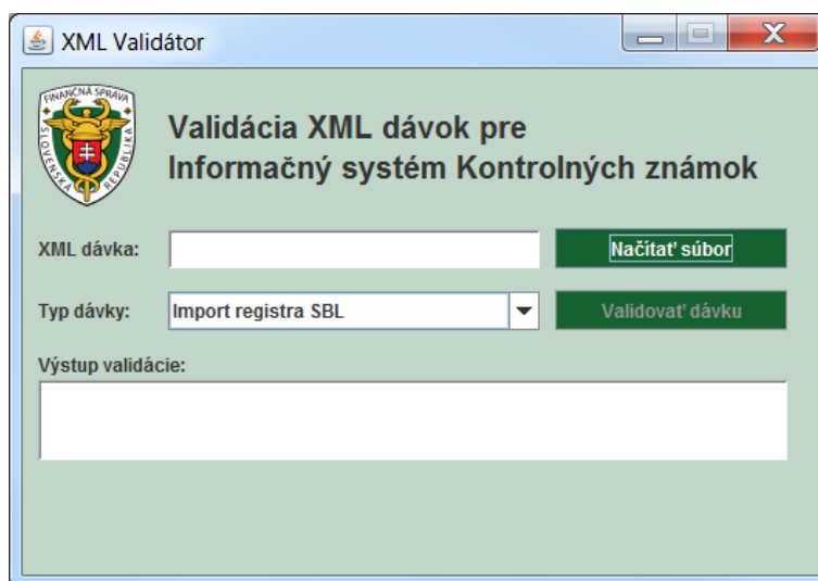
Obrázok 1. XML Validátor
